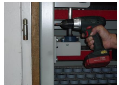
Positioniereinrichtung zum Verschrauben von Verpackungsbrettern.
